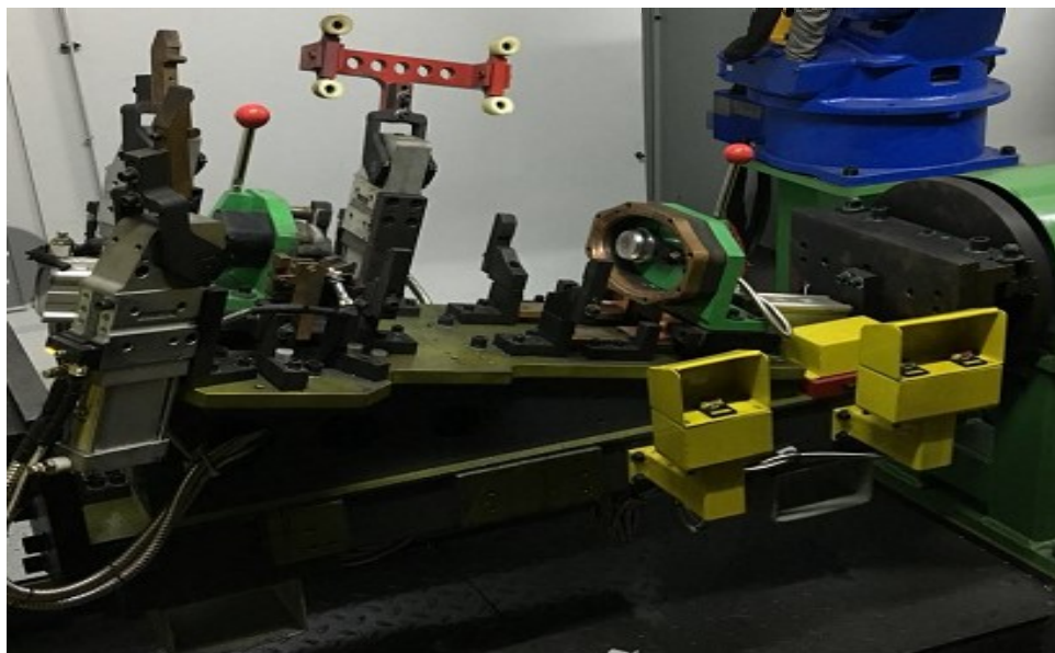
消声器焊接夹具
